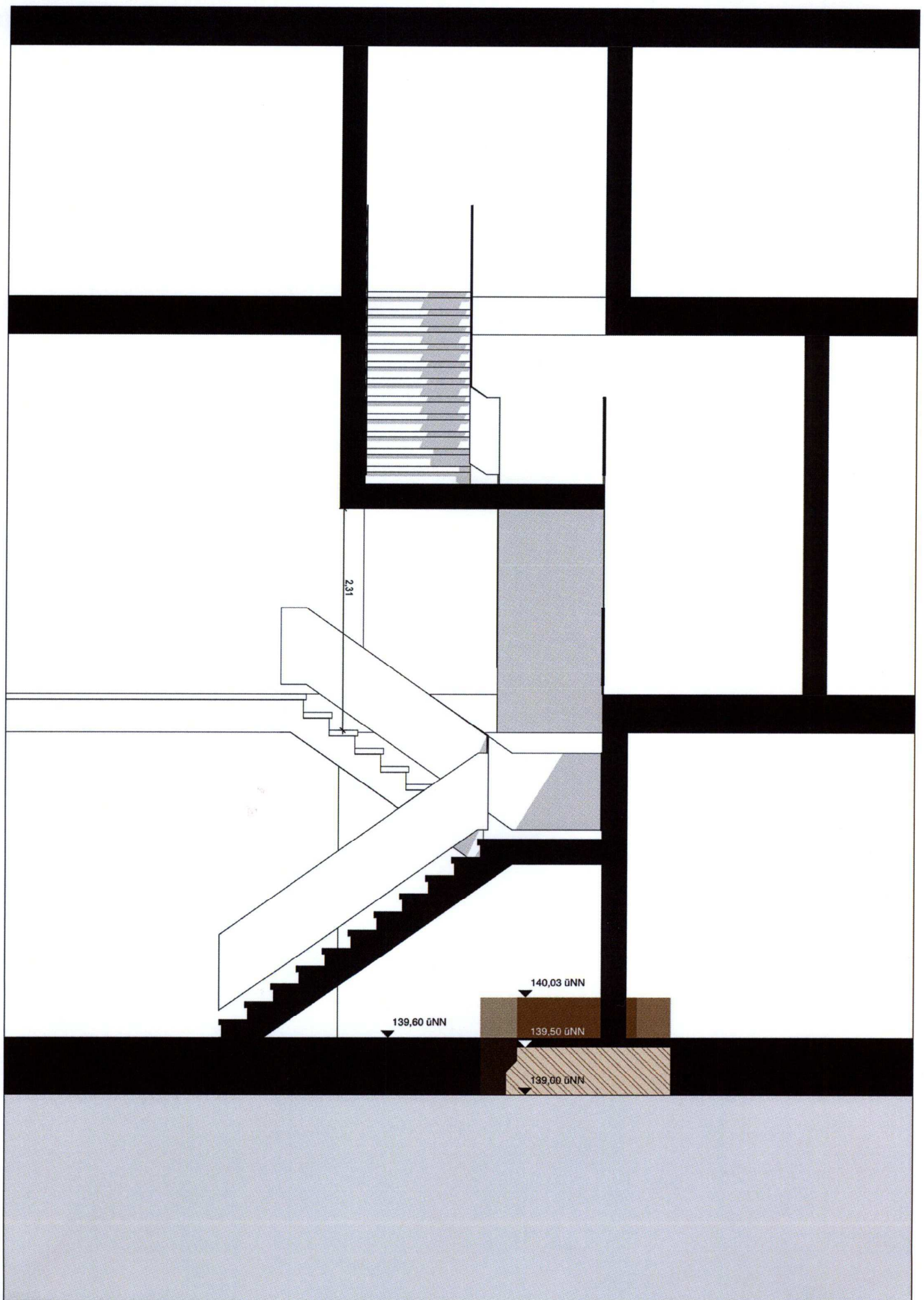
Detailschnitt Festungsmauer B - B M. 1:50
