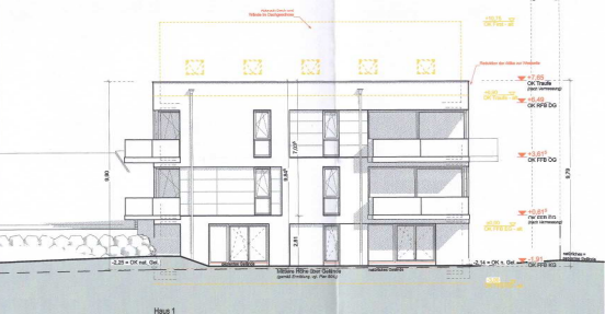
Ansicht Nordseite (Haus 1)
