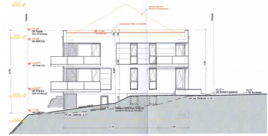
Ansicht Westseite (Haus 1)
