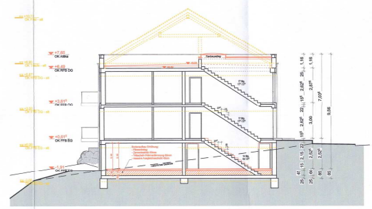
Schnitt A-A (Haus 1)
