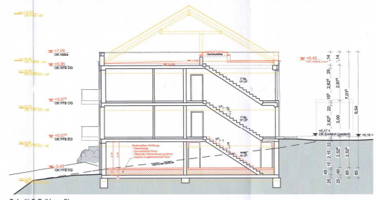
Schnitt B-B (Haus 2)
