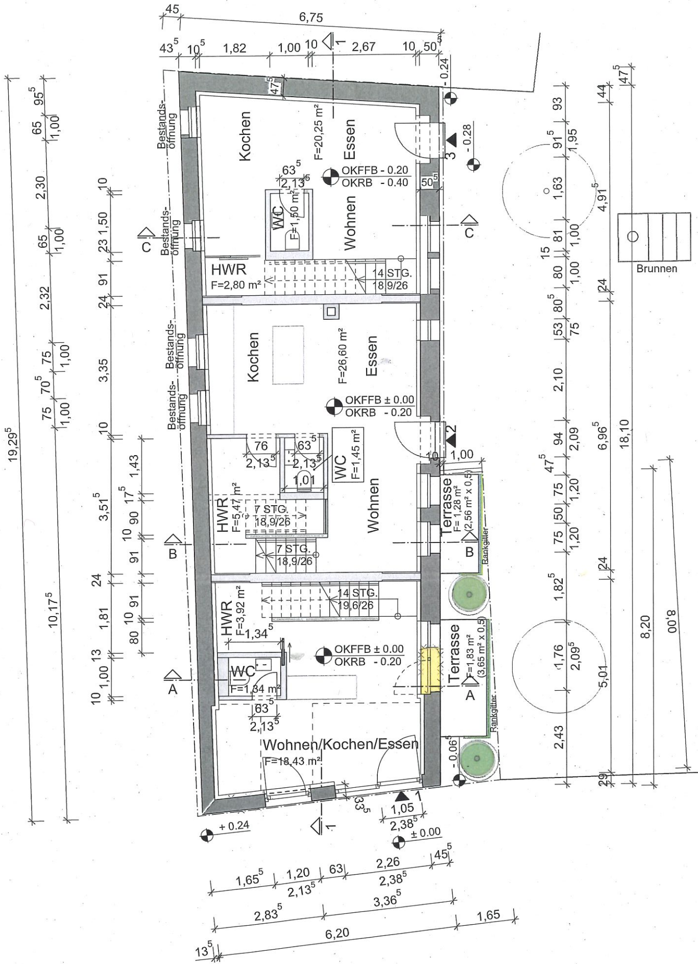
Anlage 2: Grundriss Erdgeschoss M: 1:100
