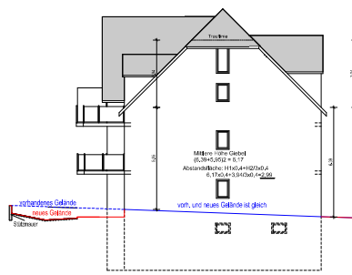
Ansicht West
