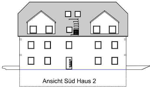
Ansicht Süd
