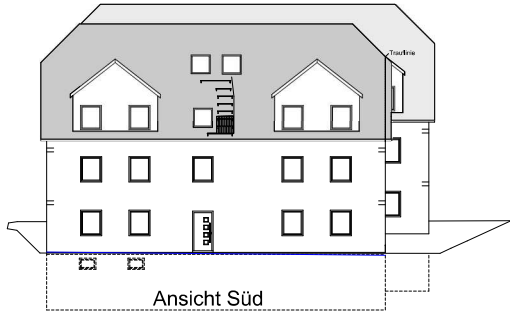
Ansicht Süd
