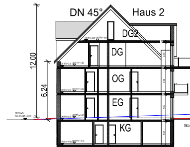
Schnitt A-A
