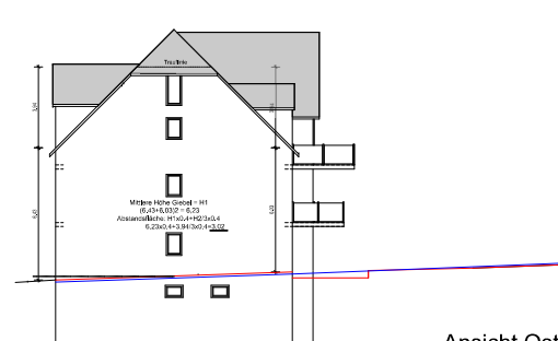
Ansicht Ost
