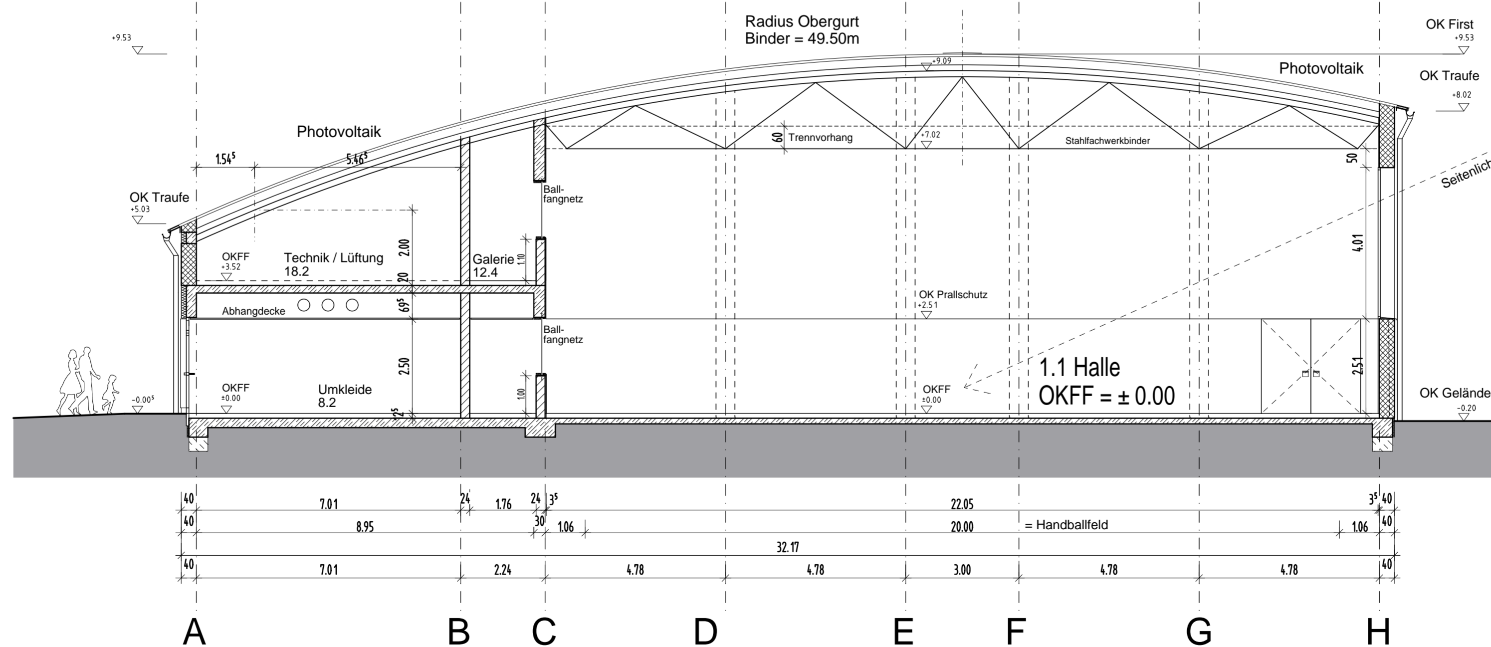
Schnitt a-a (Ansicht Wand Achse 8)
