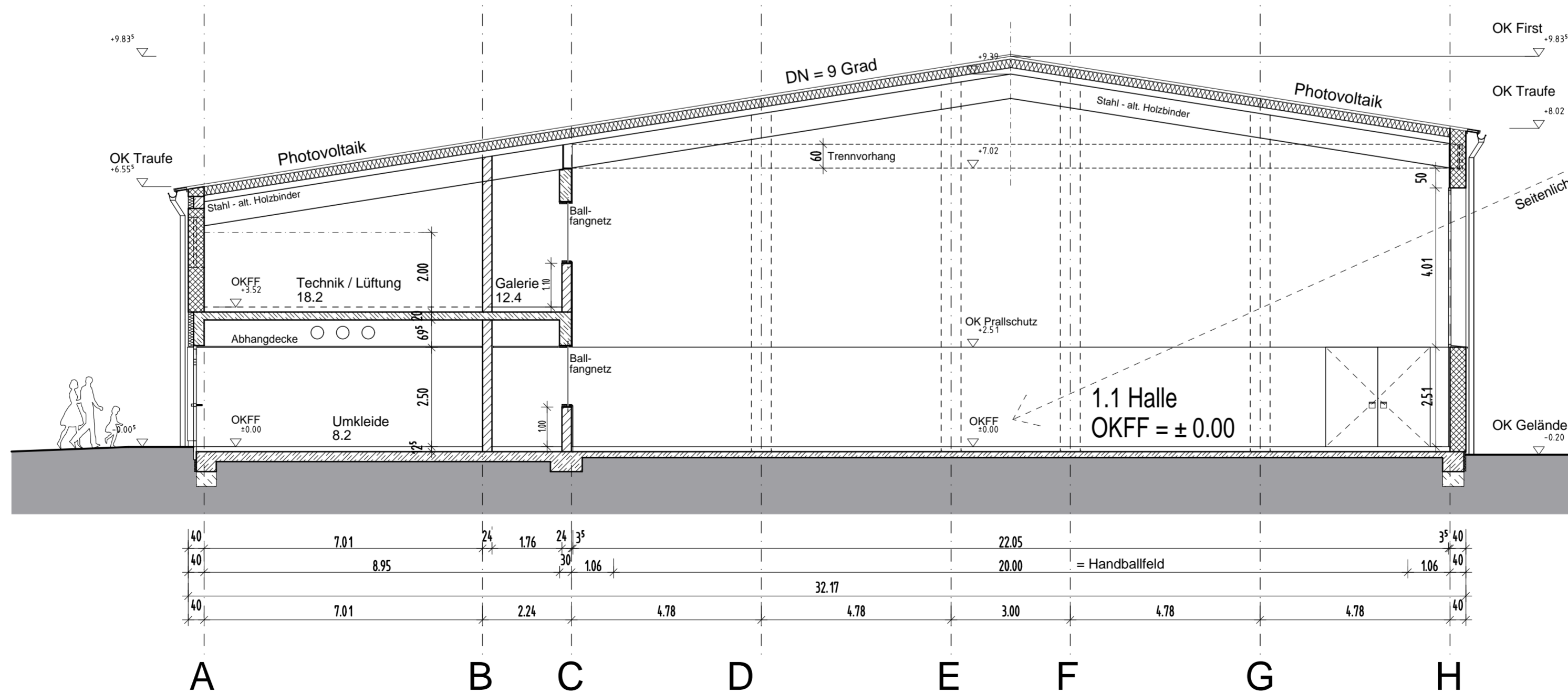
Schnitt a-a (Ansicht Wand Achse 8)
